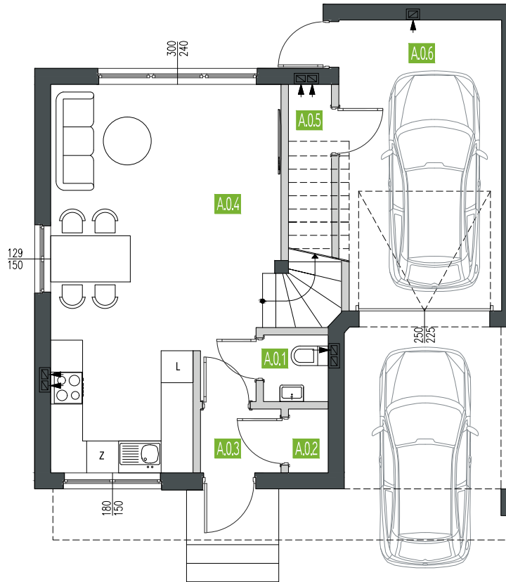
RZUT PARTERU
