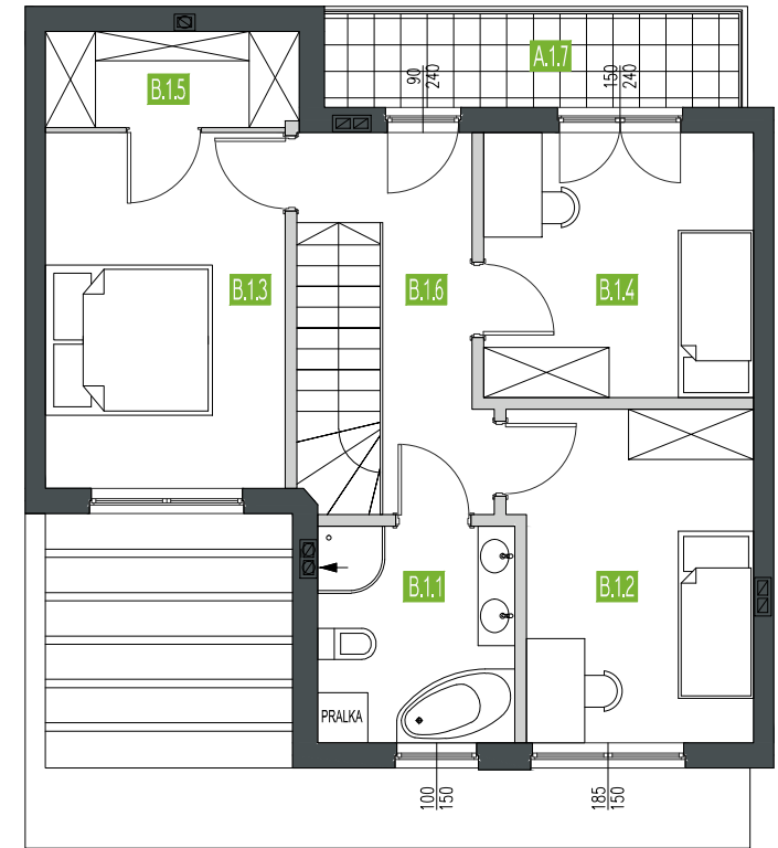
RZUT PIĘTRA
