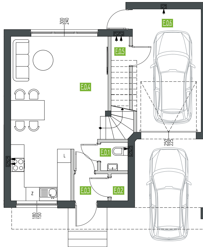
RZUT PARTERU
