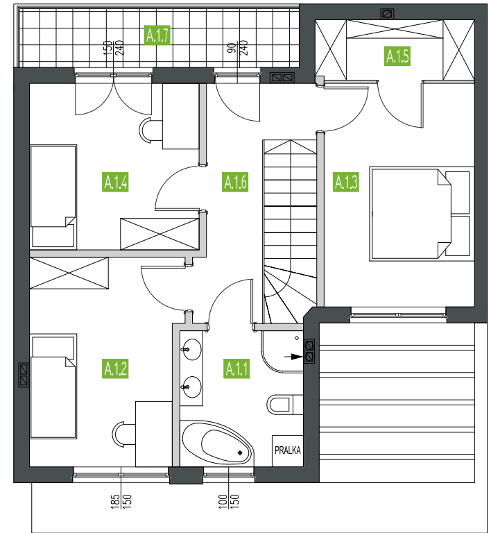
RZUT PIĘTRA
